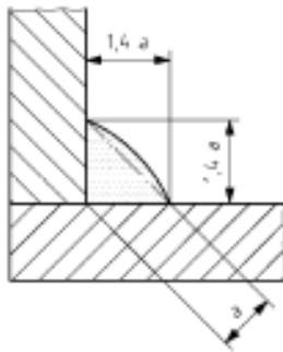
Εικόνα 1.3 Διαστάσεις εξωρραφών
