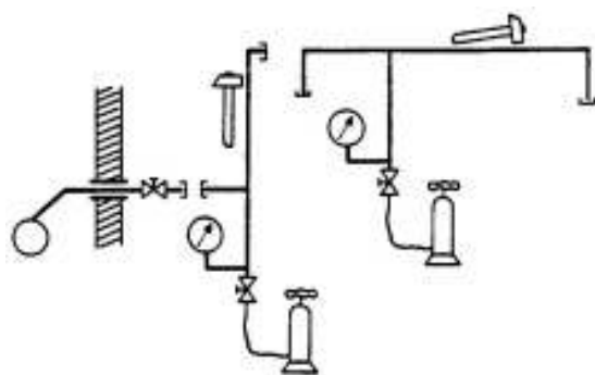
Εικόνα 10.1 Δοκιμή αντοχής
