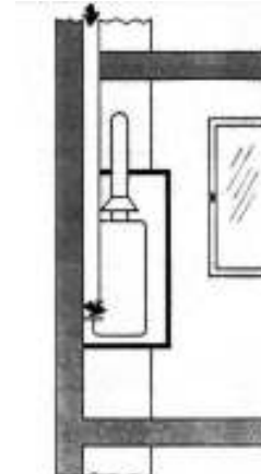
γ) τροφοδοσία αέρα με φρεάτιο επάνω από τη στέγη
