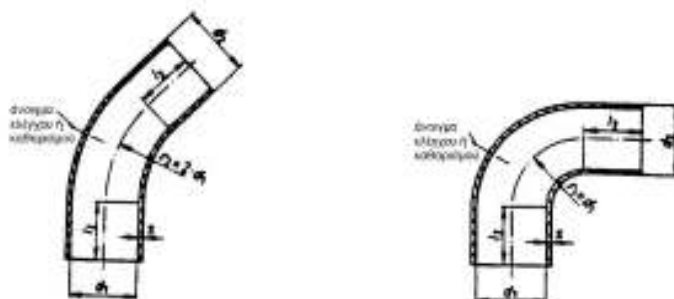
Εικ.9.4 Στοιχεία μορφής καπναγωγών από μέταλλο
