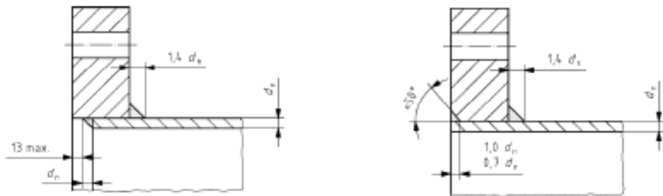
φλάντζα συγκολλητού λαιμού
